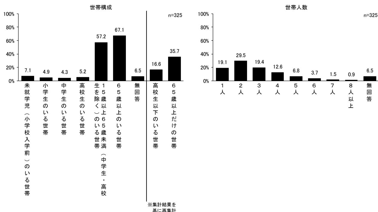
＜図表3-3-4 現在の世帯構成・人数＞
